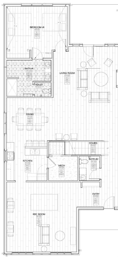
VILLA PREMIER FLOOR PLAN
